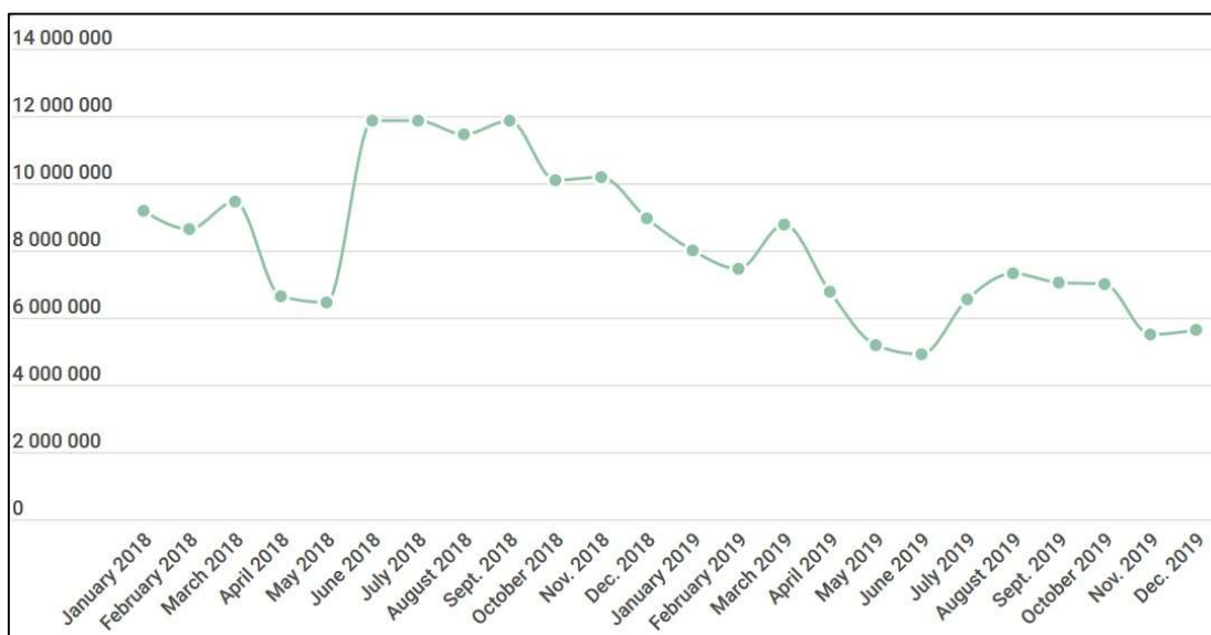
شکل شماره ۷: تعداد حملات ناموفق در سال ۲۰۱۸-۲۰۱۹
